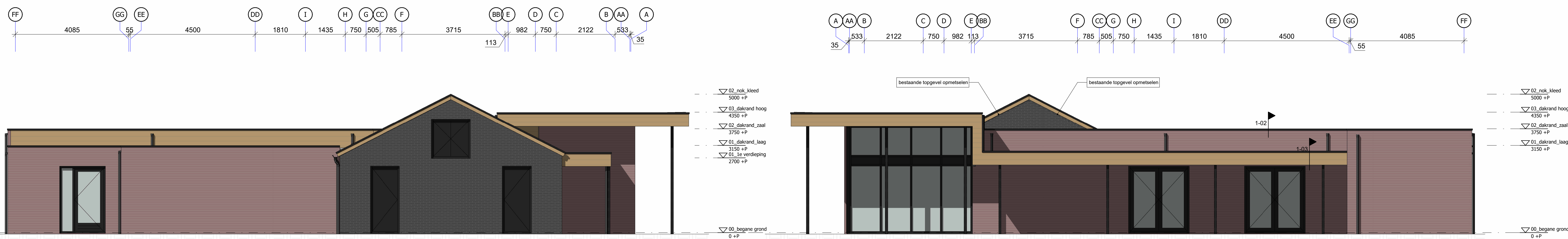
Linker zij-gevel schaal: 1 : 50
